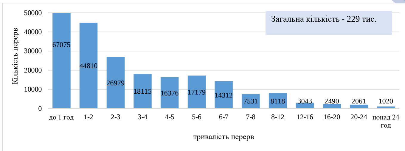
Рис. 1.29. Кількість та тривалість перерв в електропостачанні у II кварталі 2021 року (з усіх причин)
