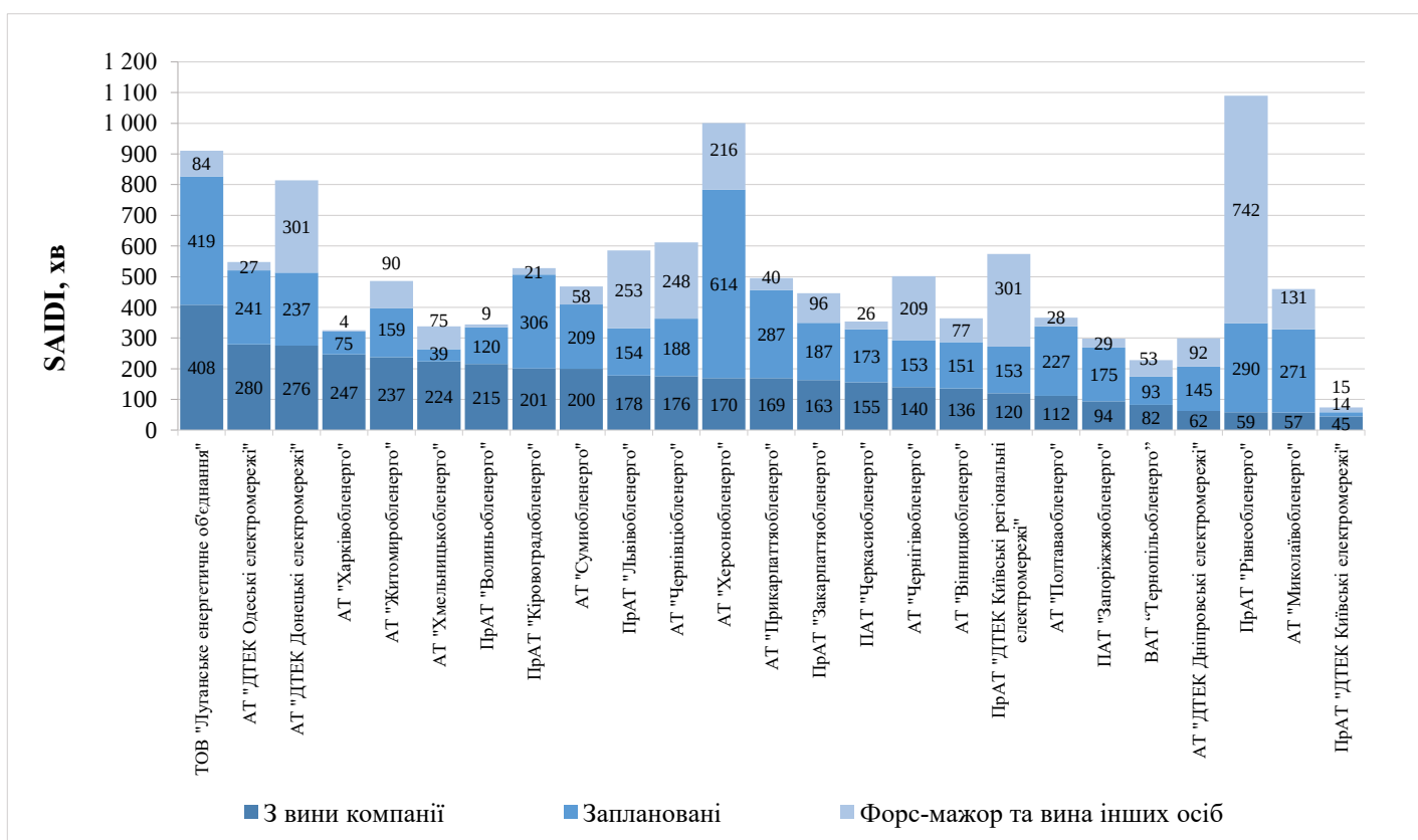
Рис. 1.28. Показники SAIDI у II кварталі 2021 року
